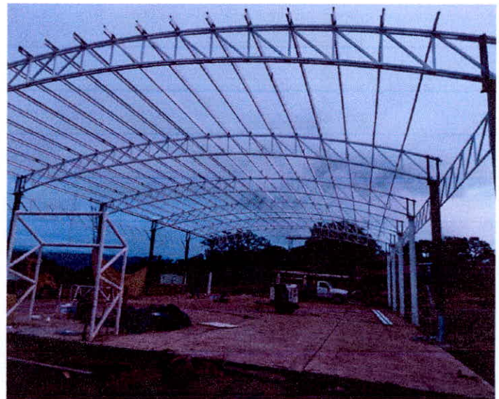
CONSTRUCCIÓN DE DOMO
