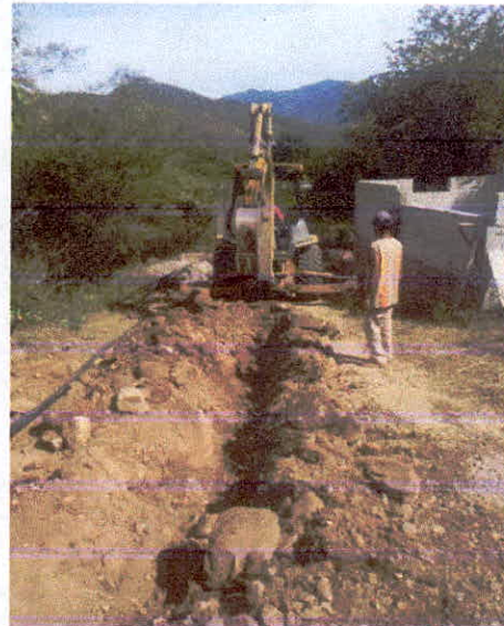
EXCAVACIÓN DE ZANJA PARA RECIBIR TUBERÍA
