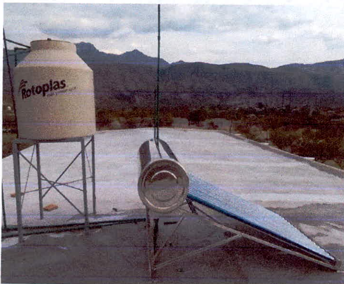
INSTALACIÓN DE CALENTADORES SOLARES
