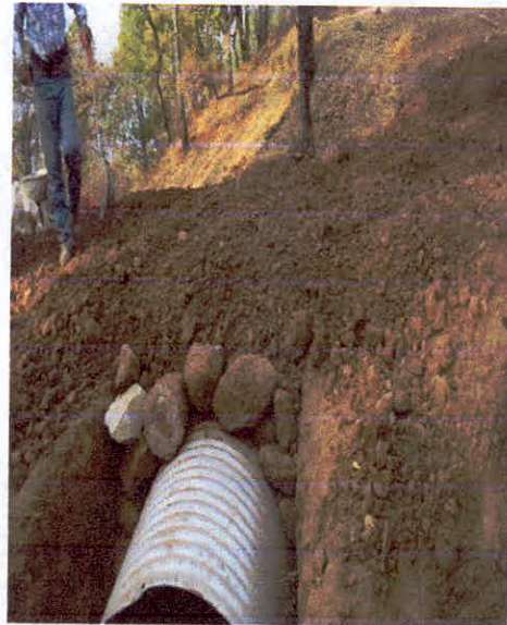
REVESTIMIENTO DE CAMINO CON MATERIAL DE BANCO Y OBRAS DE DRENAJE
